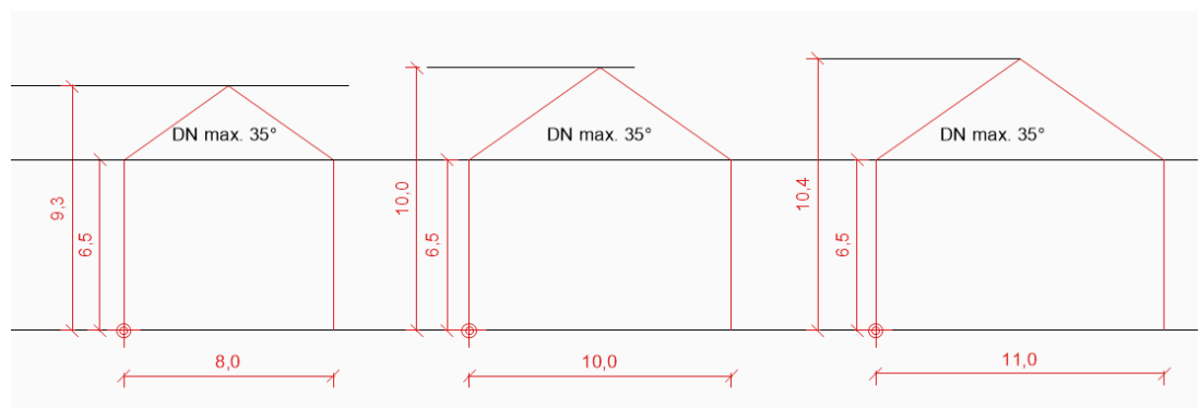
Abb. 20 Beispielschnitte für mögliche Gebäudequerschnitte bei max. Dachneigung 35^\circ
