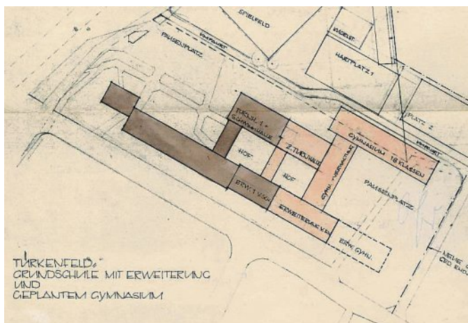
Planstudie für ein 18-klassiges Gymnasium von 1971
